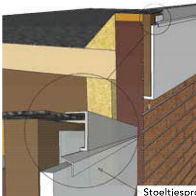
Detail 250.66 Boeideel renovatie*
