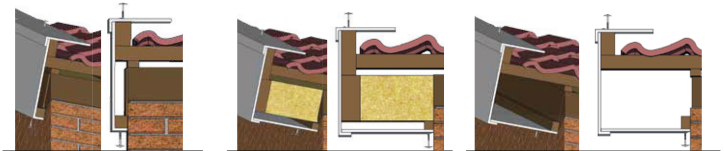
Detail 250.63 Windveer met dekker*
