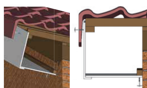
Detail 250.65A Dakoverstek met eindgevelpan*
