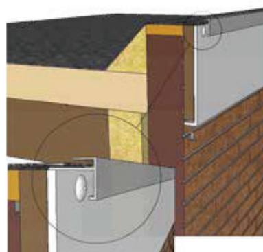
Detail 250.66 Boeideel nieuwbouw*
