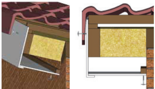
Detail 250.65 Dakoverstek met eindgevelpan*
